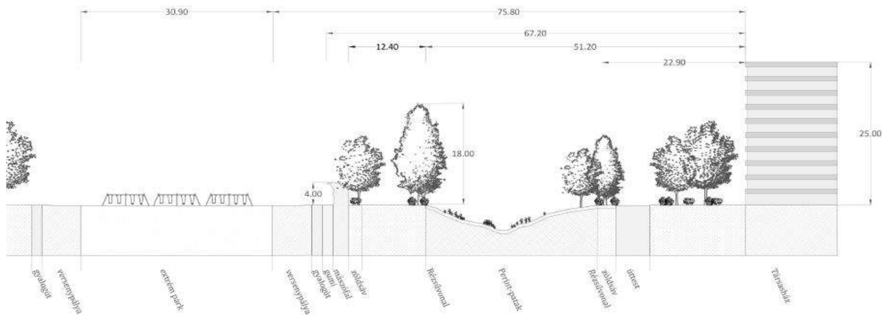
A-A metszet
